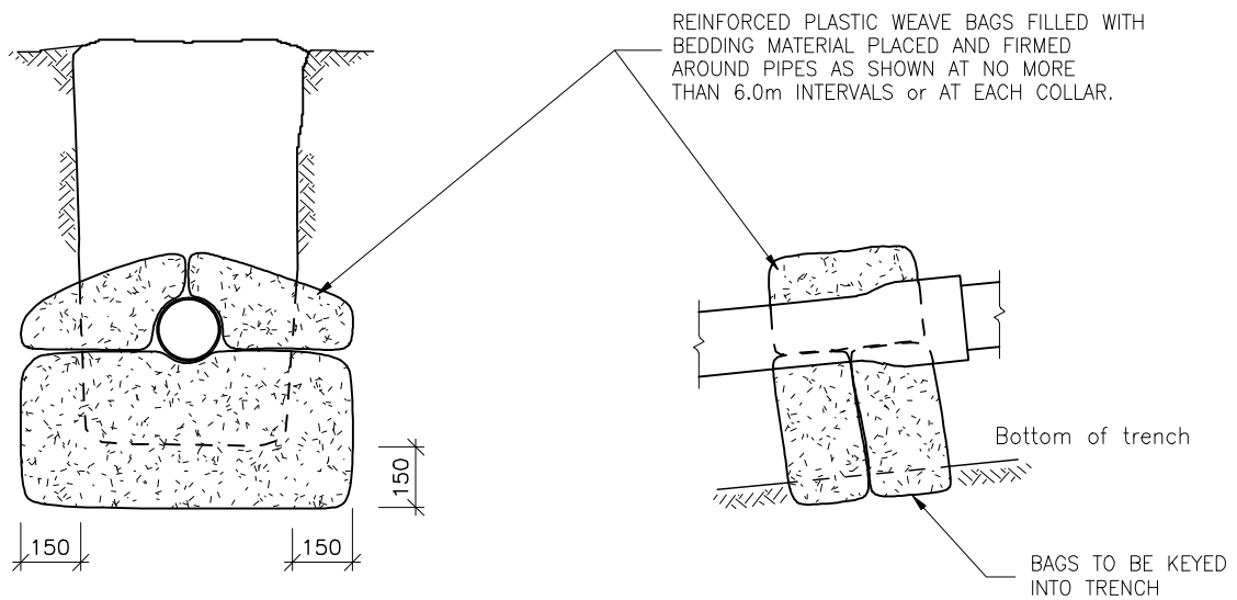
PVC & PE PIPES AT 10-20%
