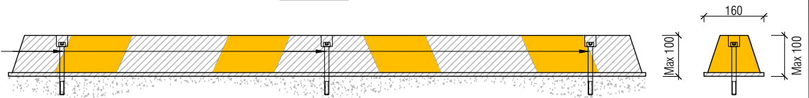
ELEVATION
