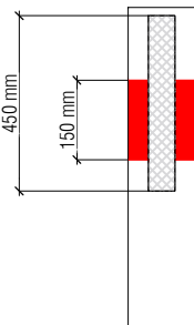
TYPE A: WHITE RETROREFLECTOR
