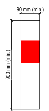
TYPE B: NO RETROREFLECTOR
